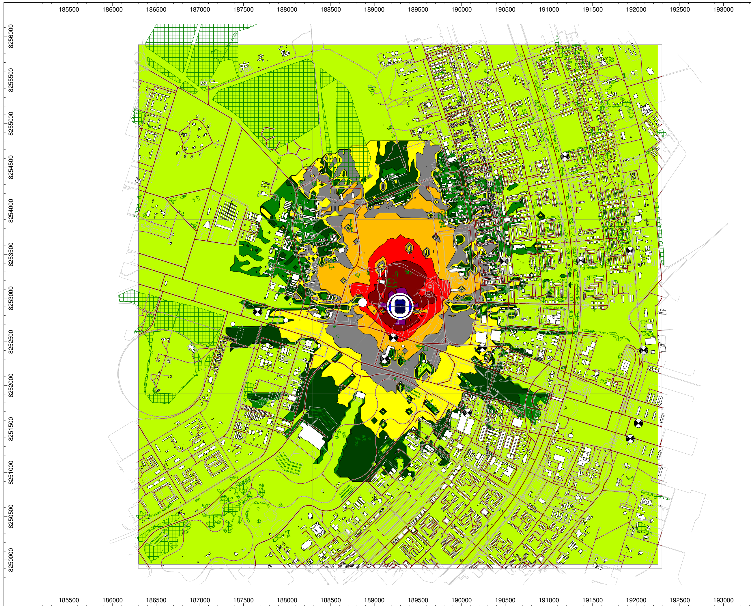
FIGURA 21 AID ESTÁDIO NACIONAL DE BRASÍLIA PALCO SUL (100 dBA) SHOW ISOLADO NÍVEL DE SEGURANÇA LIMITE NOTURNO
